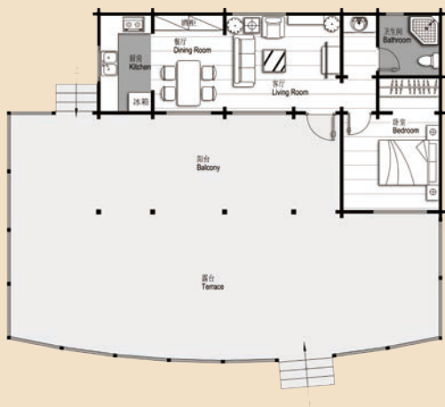
首层平面图 1:100
